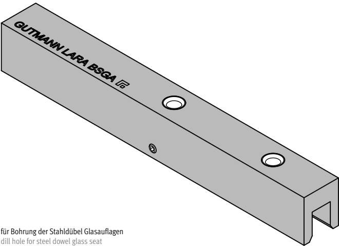
für Bohrung der Stahldübel Glasauflagen for drill hole for steel dowel glass seat
