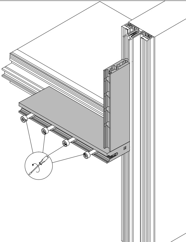
Glasauflager im horizontalen Bereich mit 4 Stück Schrauben 5,5 x 38 mm in den Schraubkanal des Riegelprofils verschrauben. Bolt the glass seat in the horizontal area with 4 screws 5.5 x 38 in the screw channel of the transom profile.
