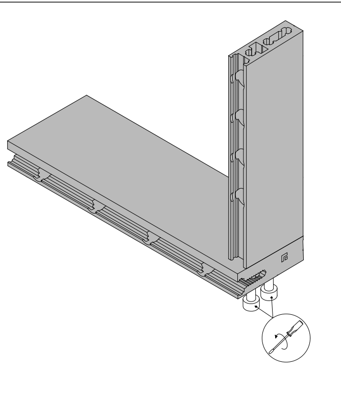
Kreuzadapter und Glasauflage mit 2 Stück Zylinder- kopfschrauben 5,5 x 38 mm (im Set enthalten) verschrauben. Screw the cross adapter and glass seat with two cylinder head screws 5,5 x 38 mm (included in set).
