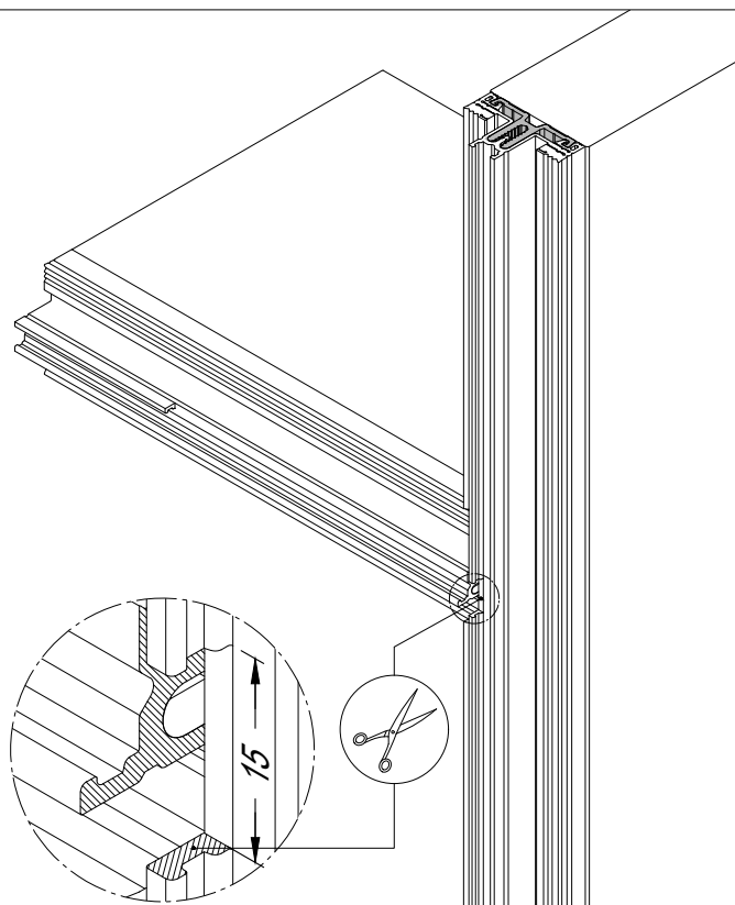
Pfostendichtung im Bereich der horizontalen Glasauflage 15 mm ausklinken. Notch the mullion gasket in the horizontal area 15 mm.
